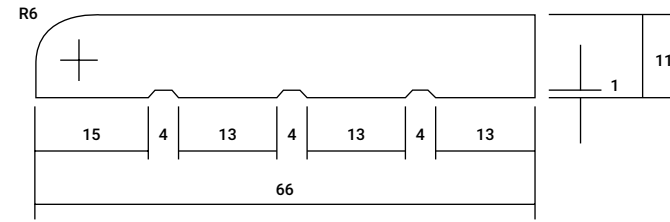
PENCIL ROUND AS15 66mm x 11mm
