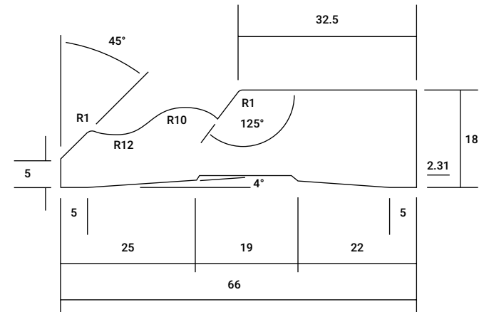
COLONIAL AS2 66mm x 18mm
