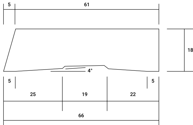
BEVEL AS3 66mm x 18mm
