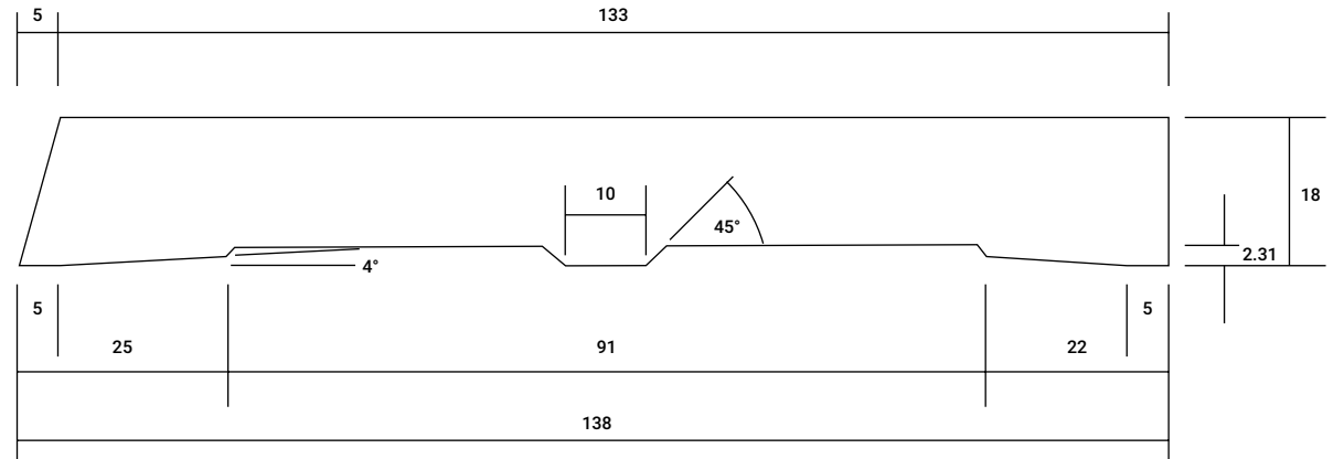
BEVEL AS3 138mm x 18mm
