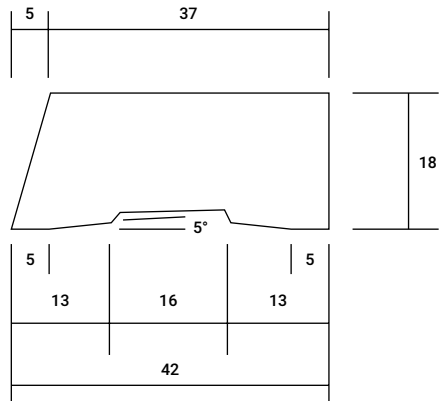
BEVEL AS3 42mm x 18mm
